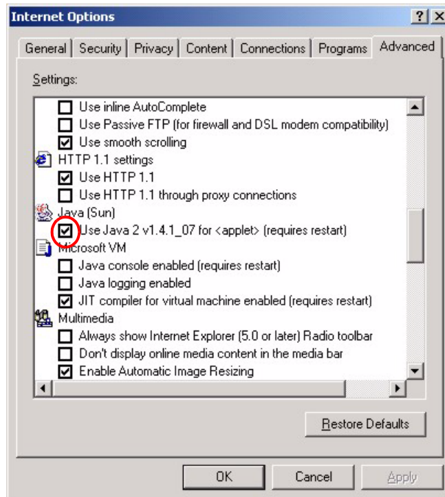
Figure 122 Java (Sun)
